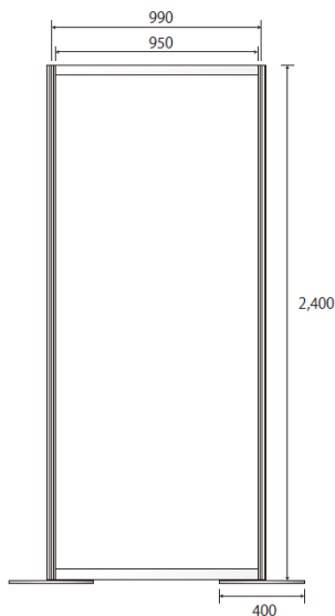
立面図
